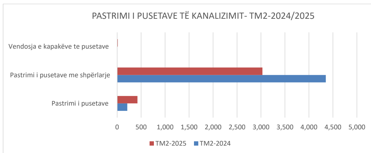
Diagrami nr.4 - Pastrimi i pushtave të kanalizimit – TM2-2024/2025
